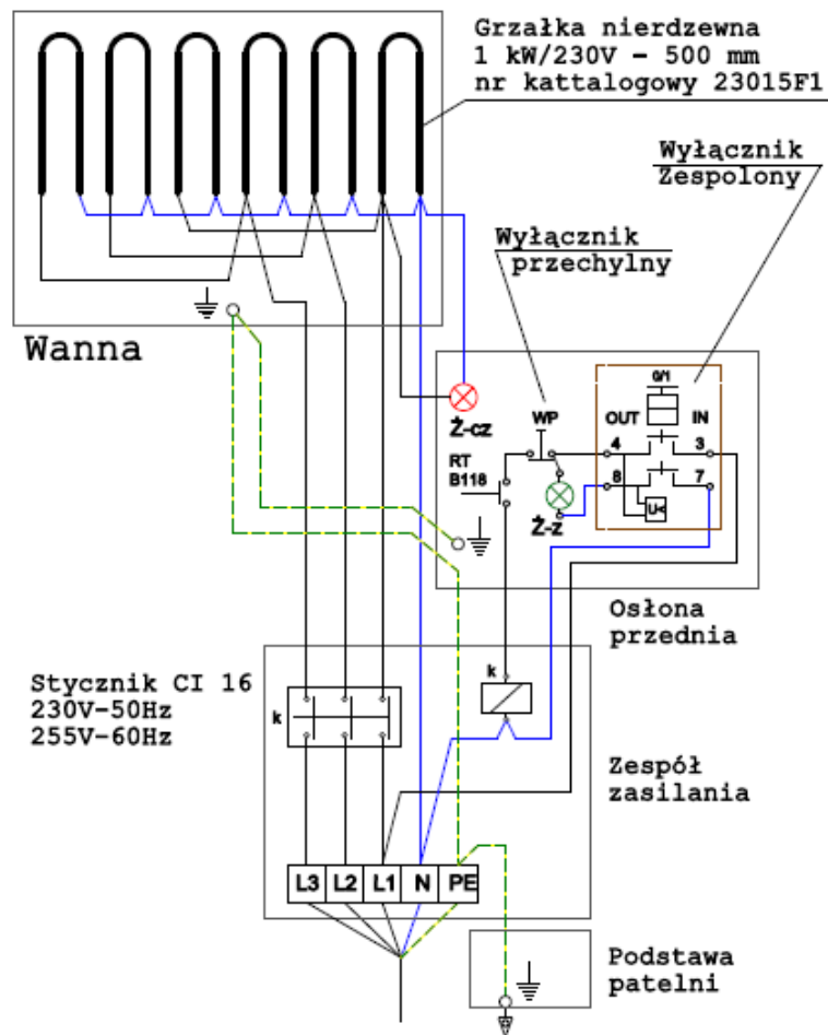
Rysunek 5 Schemat elektryczny
